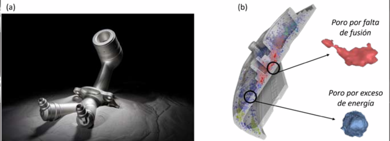
Fig. 2. (a) Inyector de combustible LEAP de GE Aerospace [1]. (b) TC de un componente industrial, con poros detectados representados en distintos colores según su volumen [2].
